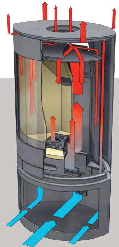
Weergave van de luchtstromen in de haardkachel
